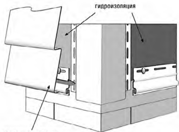
зашелкните сайдинг в стартовую полосу и сдвиньте к стойке угла
