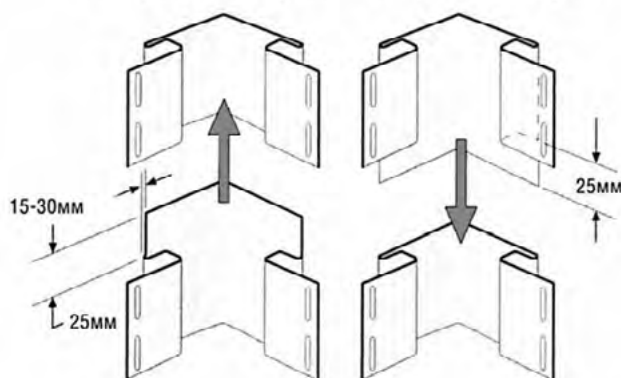
1-й вариант стыковки углов
